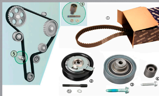
Image 1: Schéma d'entraînement 1.9 TDI/SDI et contenu du Kit 5549173/ 5549170
