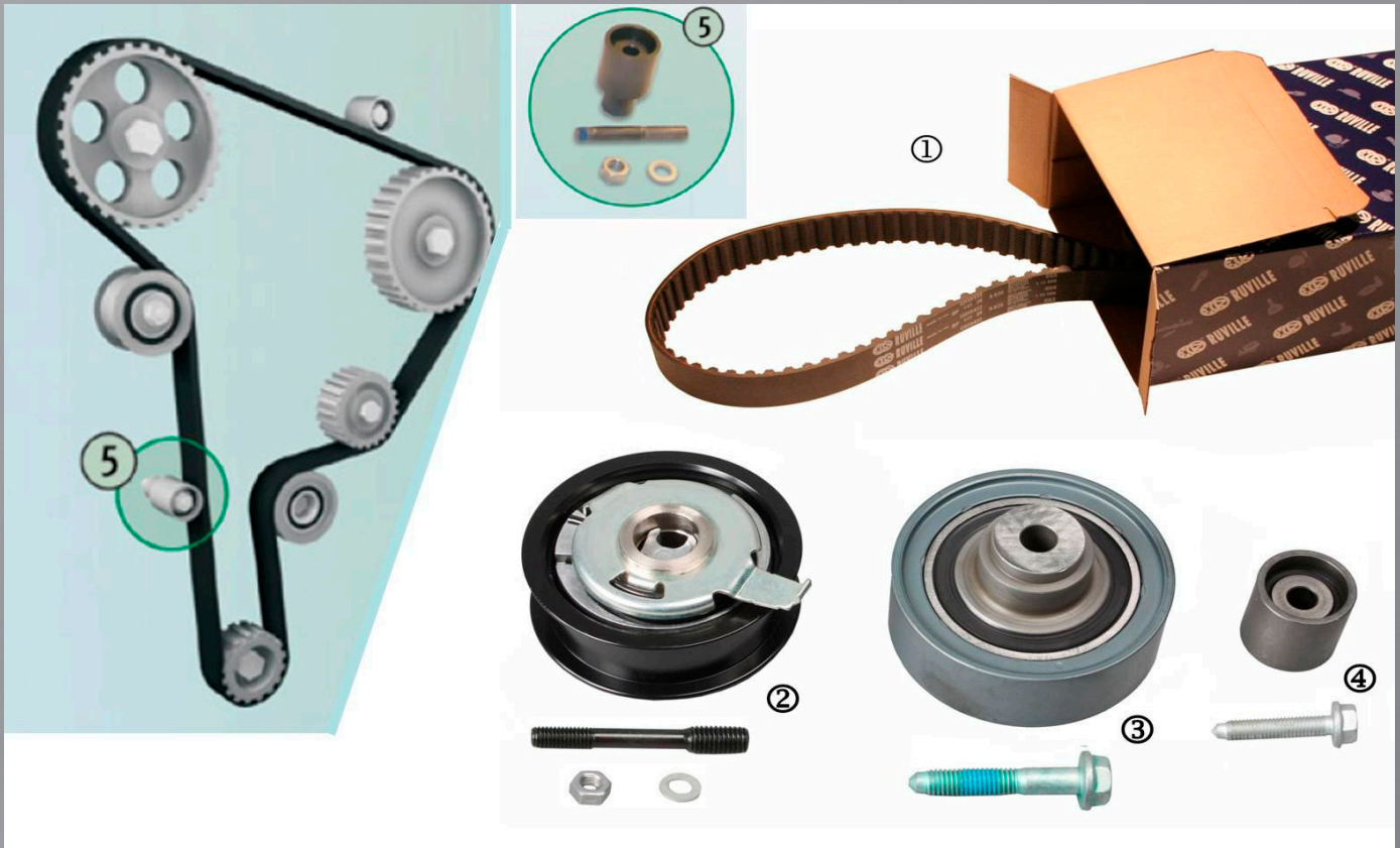
Image 1: Schéma d'entraînement 1.9 TDI/SDI et contenu du Kit 5549173/ 5549170
