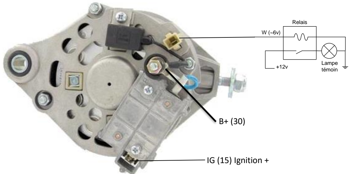
013482 : Alternateur sans diode d'excitation
