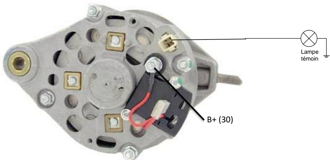
013483 : Alternateur avec diodes d'excitation
